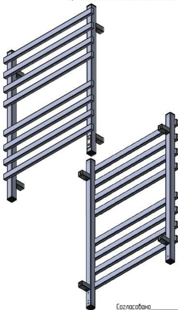
Электрический полотенцесушитель ДВИН Серии NEO МОДЕЛЬ N PLAZA NEO 800x500
