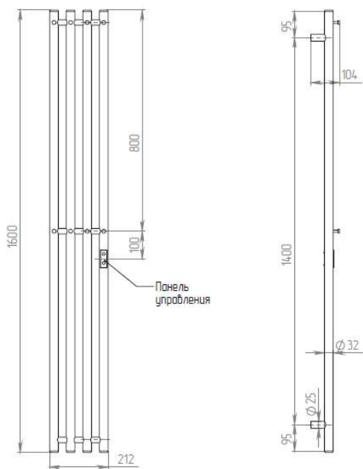
Электрический полотенцесушитель ДВИН Модель X-4 нео -1400x180
