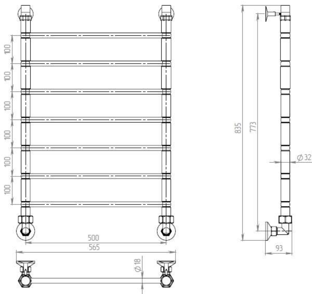
Водяной полотенцесушитель ДВИН Модель Bubble1 800x500
