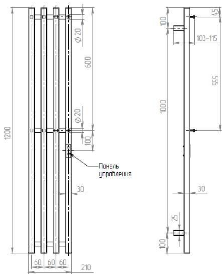
Электрический полотенцесушитель ДВИН Модель X-4 plaza neo -1200x180
