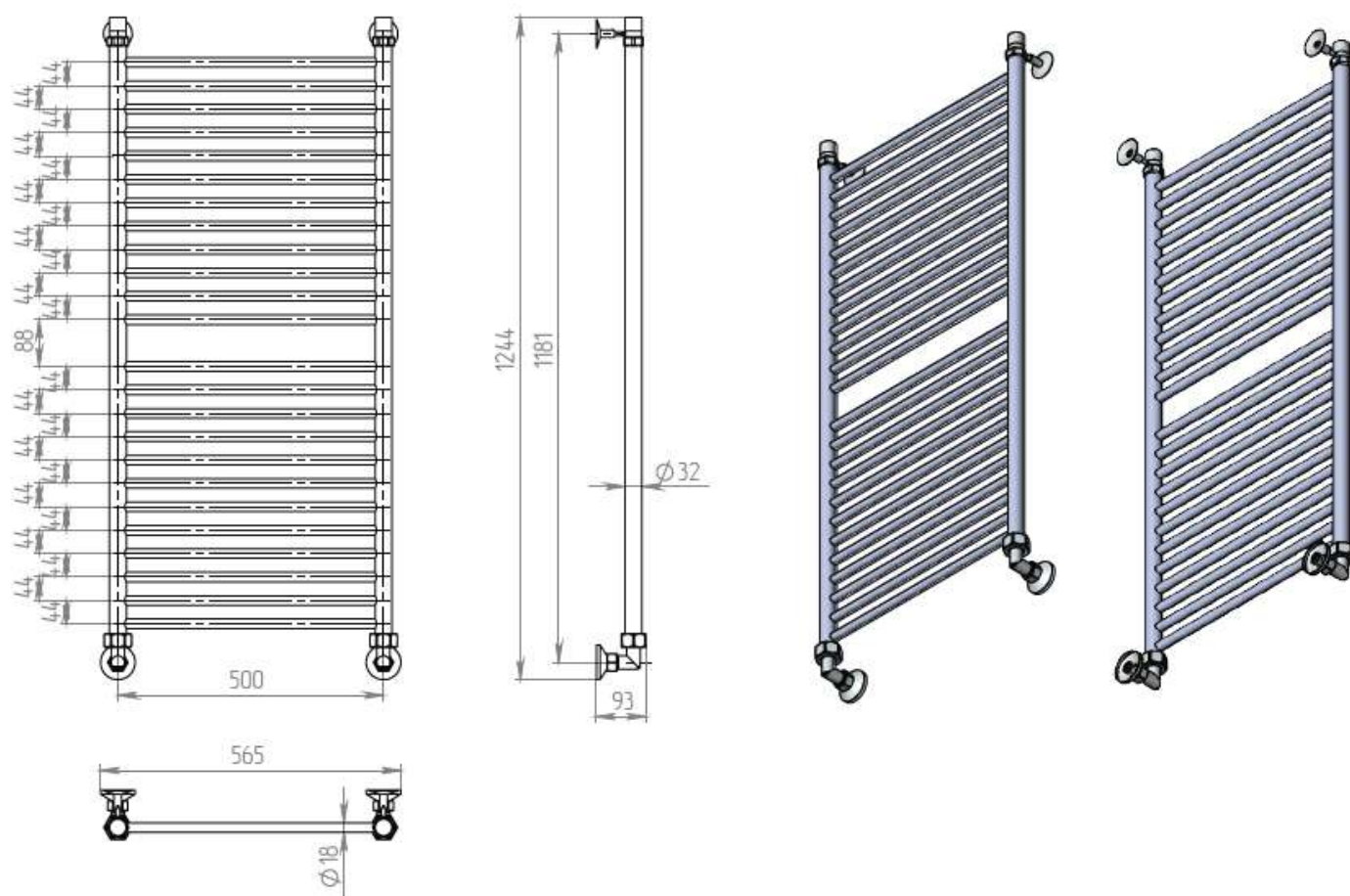
Водяной полотенцесушитель ДВИН Модель S 1200x500
