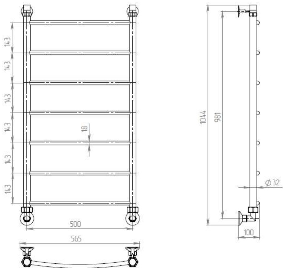
Водяной полотенцесушитель ДВИН Модель R 1000x500
