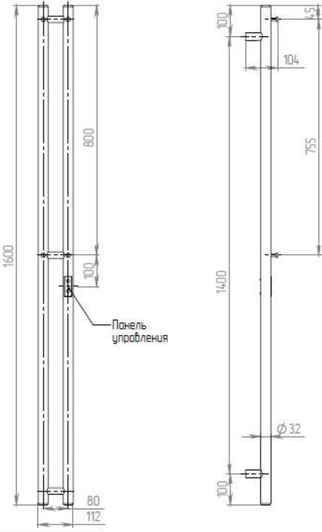
Электрический полотенцесушитель ДВИН Модель X-2 нео -1600x80
