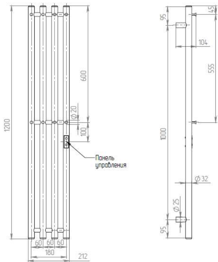
Электрический полотенцесушитель ДВИН Модель X-4 нео -1200x180
