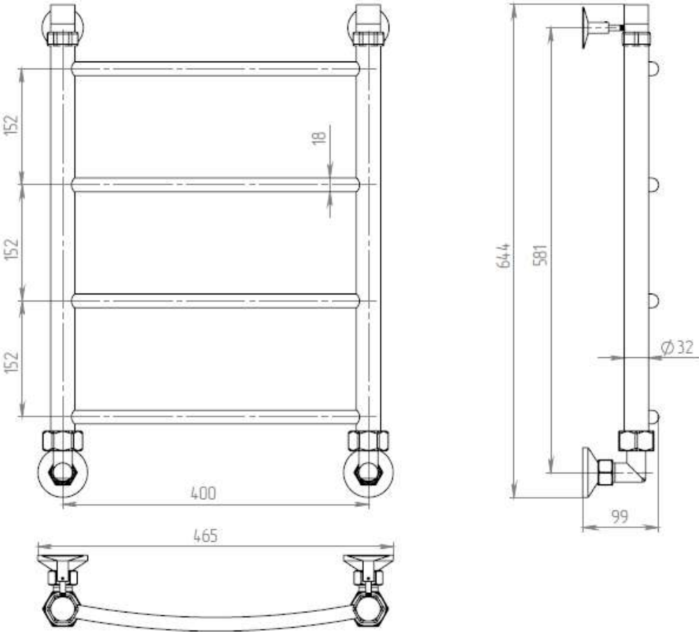
Водяной полотенцесушитель ДВИН Модель R 600x400
