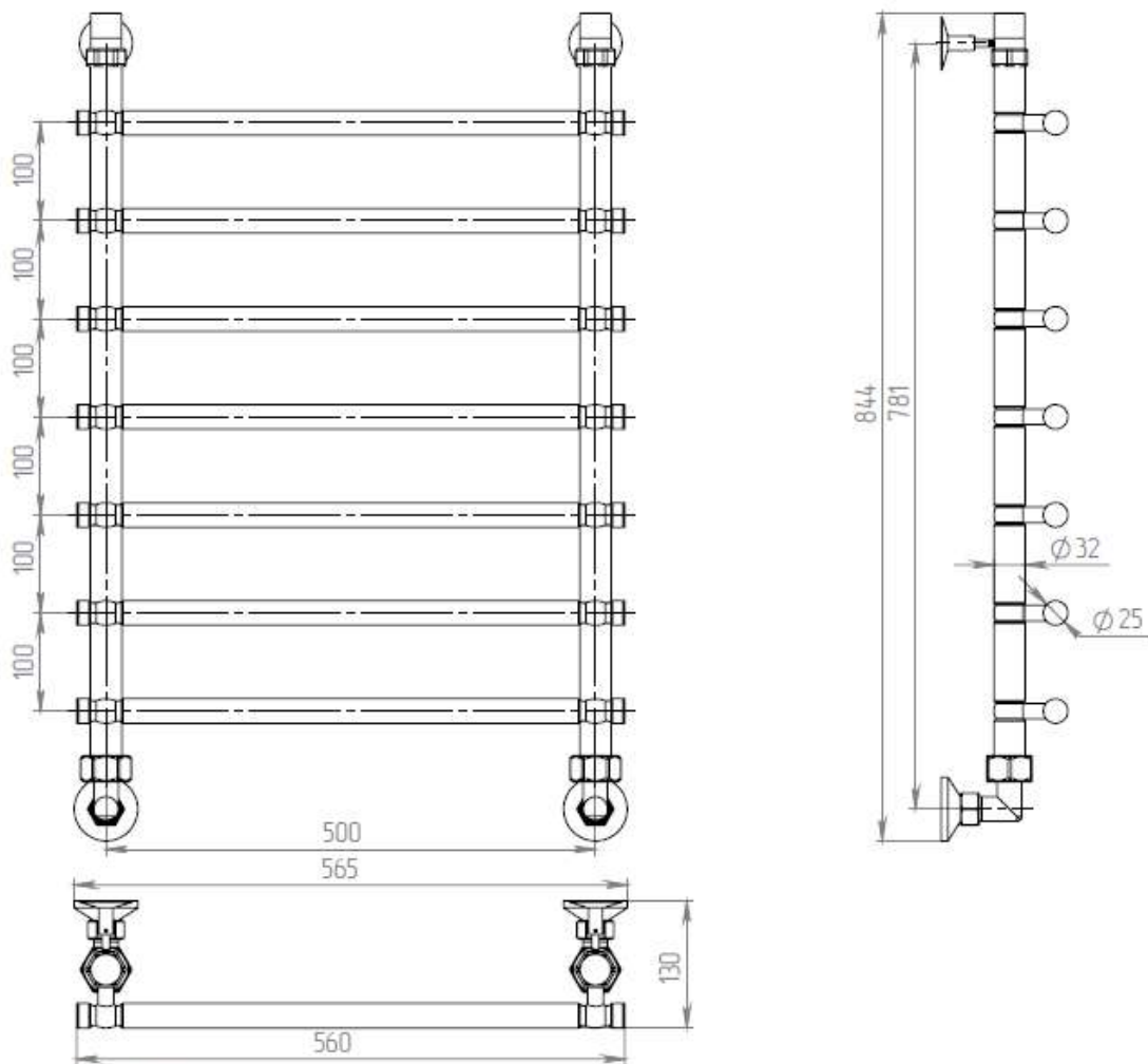
Водяной полотенцесушитель ДВИН Модель Bubble3 800x500
