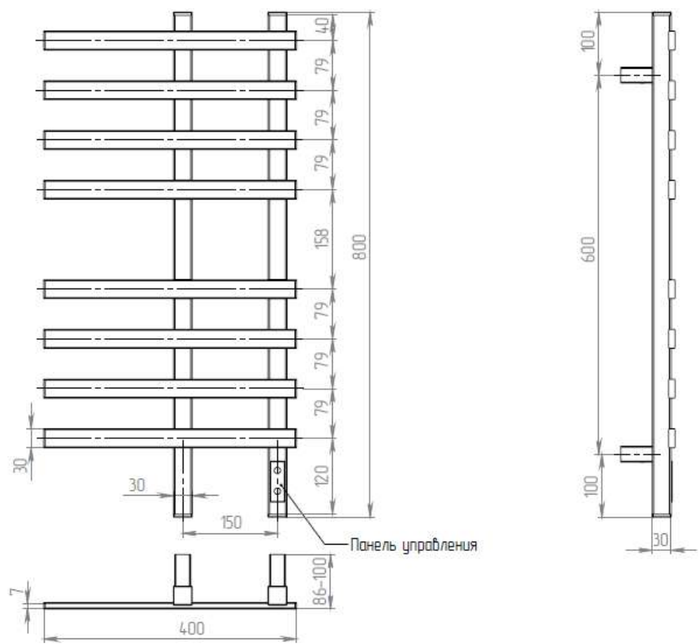
Электрический полотенцесушитель ДВИН Модель LX PLAZA NEO 800x400
