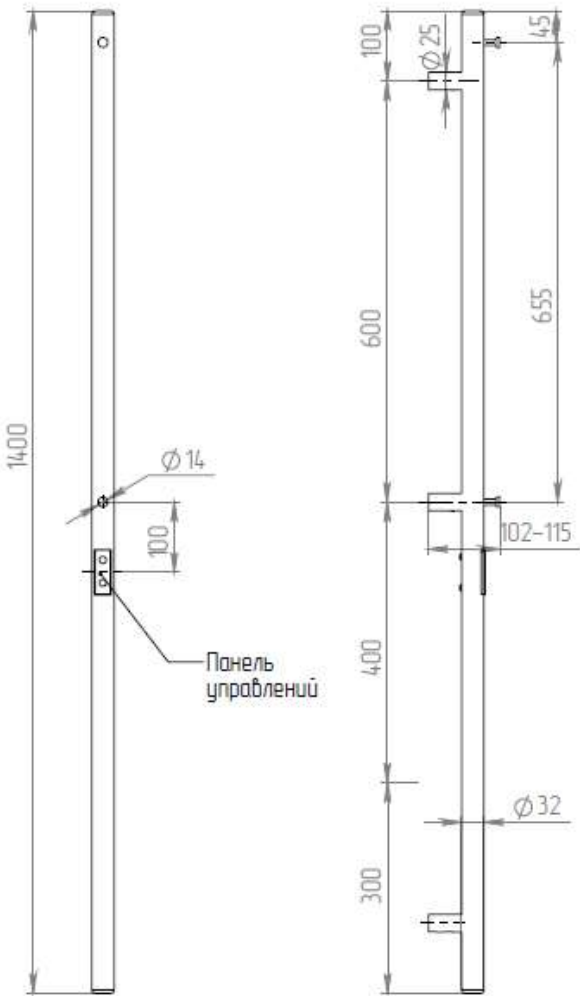
Электрический полотенцесушитель ДВИН Модель X-1 нео -1400х32
